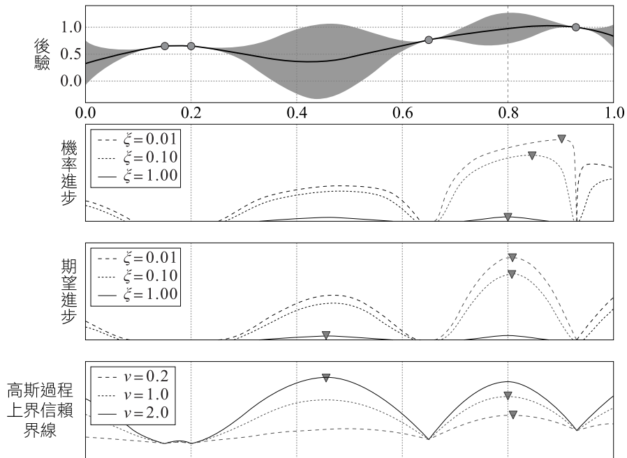
圖 F.9 機率進步、期望進步與信賴界限的比較 (Brochu et al., 2010)
