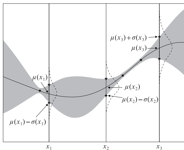
圖 F.6 高斯過程的函數平均數與變異數 (Brochu et al., 2010)
