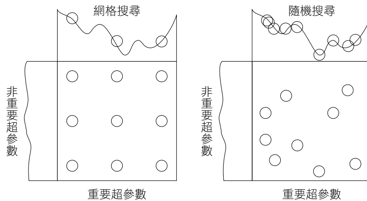
圖 F.3 網格搜尋法與隨機搜尋法 (Feurer and Hutter, 2019)
