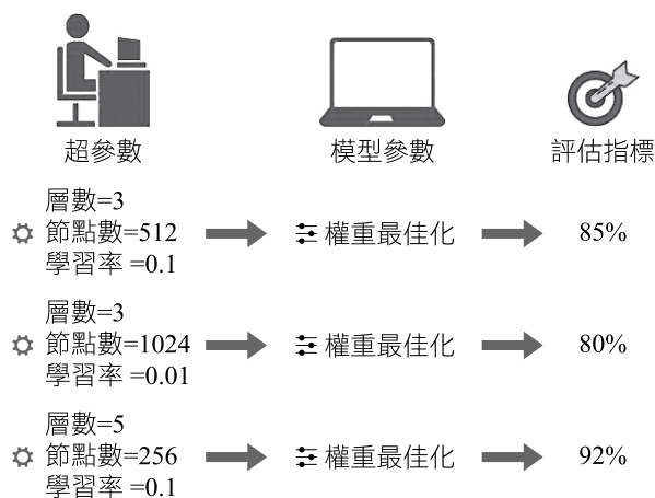
圖 F.2 超參數最佳化於類神經網路模型
