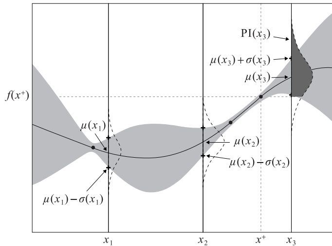
圖 F.8 機率進步的收穫函數 (Brochu et al., 2010)
