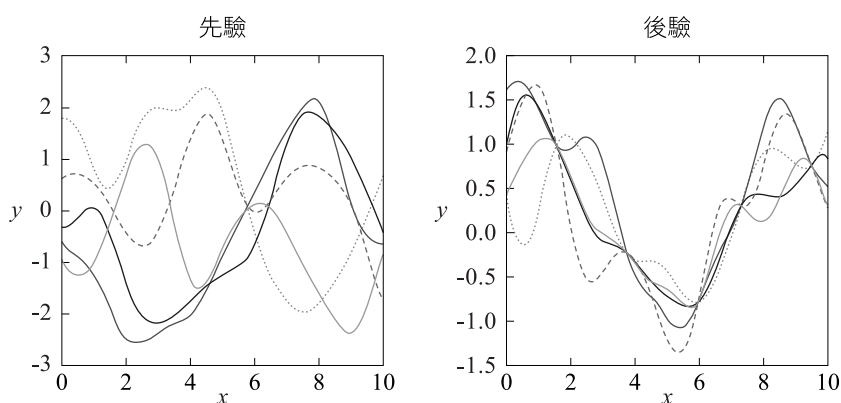
圖 F.5 高斯過程的先驗與給定五點的後驗
